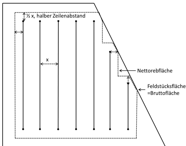
Abbildung 3: Messung der Nettoreibfläche nach der Maßnahme
